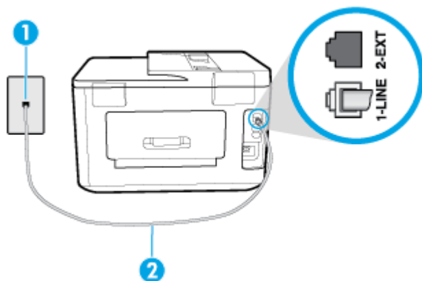
Figure 5-3 Vue arrière de l'imprimante
